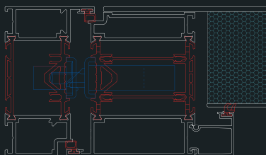
JAMB DETAIL
