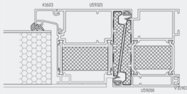
JAMB DETAIL
