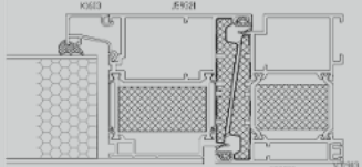
JAMB DETAIL
